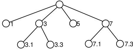
Fig. 5 OrdPath prefix scheme
