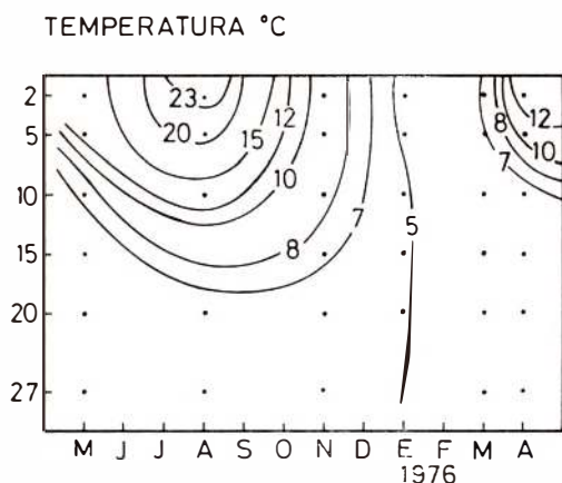
FIG. 2. — Distribución de la temperatura en función del tiempo y de la profundidad. En ésta y en sucesivas figuras los puntos negros indican las muestras estudiadas, interpolándose las isopletas.
