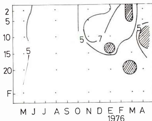
FIG. 8. — Distribución de la concentración de clorofila a en función del tiempo y de la profundidad. (El área rayada corresponde a concentraciones superiores a 8 \text{ mg/m}^3 .)
