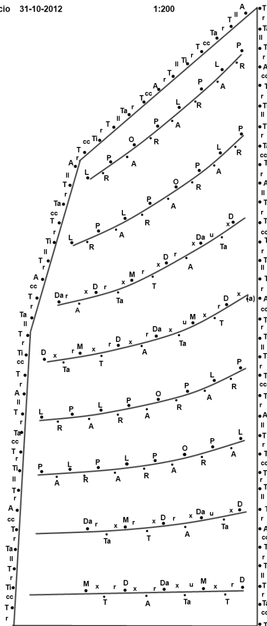
Figura 1: Diseño final de parcela agroforestal en Don Indalecio Vallejos.
