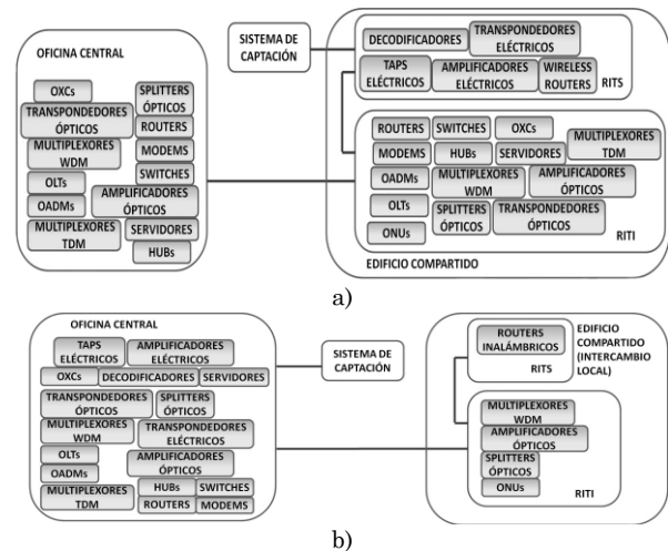
Fig. 8. Simplificación de la red: a) Distribución de la infraestructura de la red actual. b) distribución de la infraestructura de una red basada en Fi-Wi.
