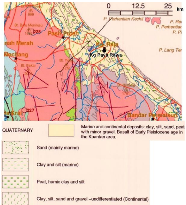
Fig. 2 Geology map of Kampung Paya Rawa, Besut. [12]
