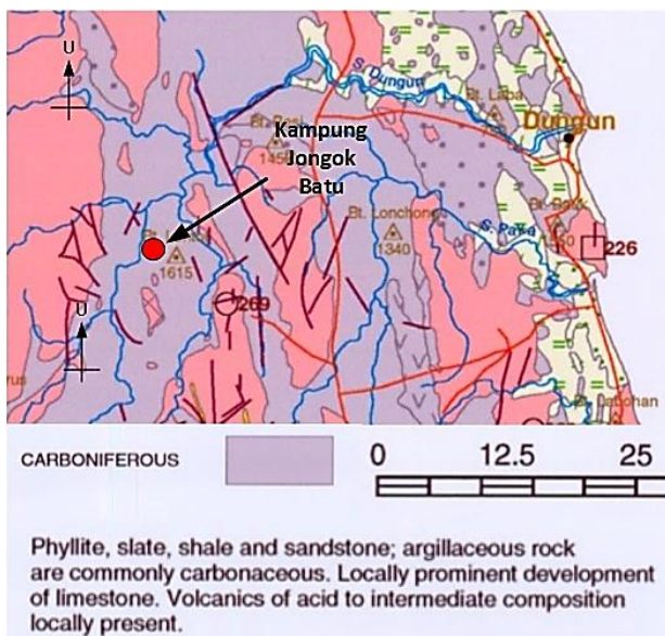
Fig.1 Geology map of Kampung Jongkok Batu, Dungun. [12].
