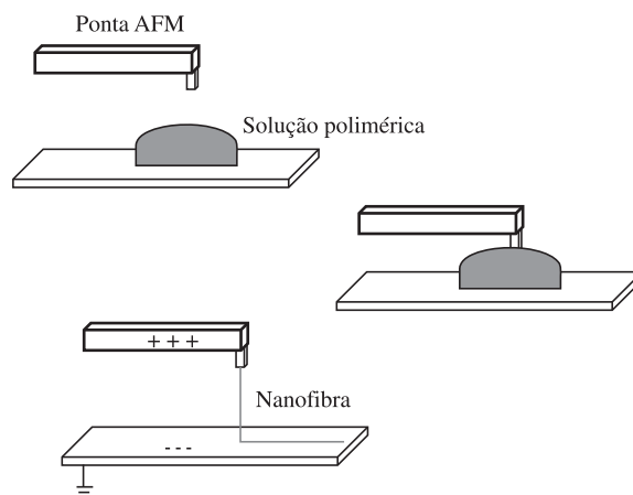
Figura 1. Representação esquemática do processo de nanoeletrofiliação baseado em microscópio de força atômica.
