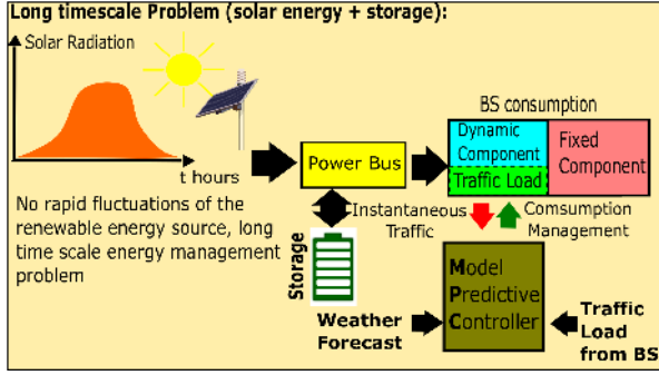
Fig. 6: MPC Scheme.
