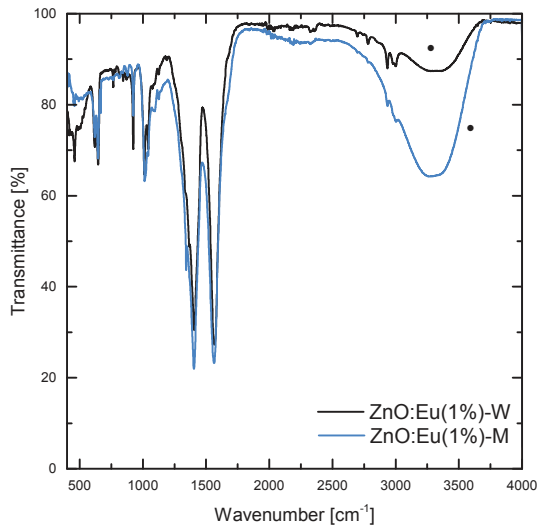
Fig. 5. FTIR spectra of ZnO:Eu(1%)-W and ZnO:Eu(1%)-M samples.
