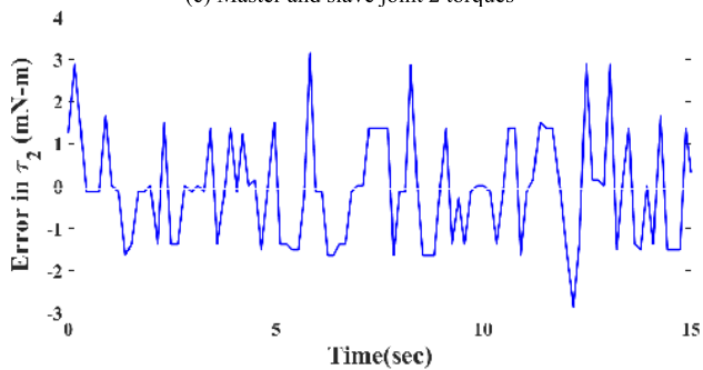
(d) Error in joint 2 torques
