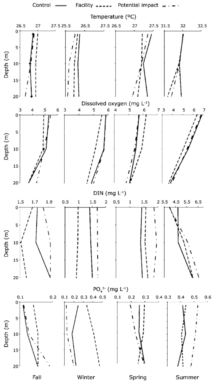
Figure 2. Temperature, dissolved oxygen, dissolved inorganic nitrogen (DIN) and phosphates (PO 4 3- ) in the water column at the control, facility and potential impact stations, for an annual cycle (2014-2015) / Temperatura, oxígeno disuelto, nitrógeno inorgánico disuelto (DIN) y fosfatos (PO 4 3- ) en la columna de agua en las estaciones de control, jaulas flotantes e impacto potencial para un ciclo anual (2014-2015)
