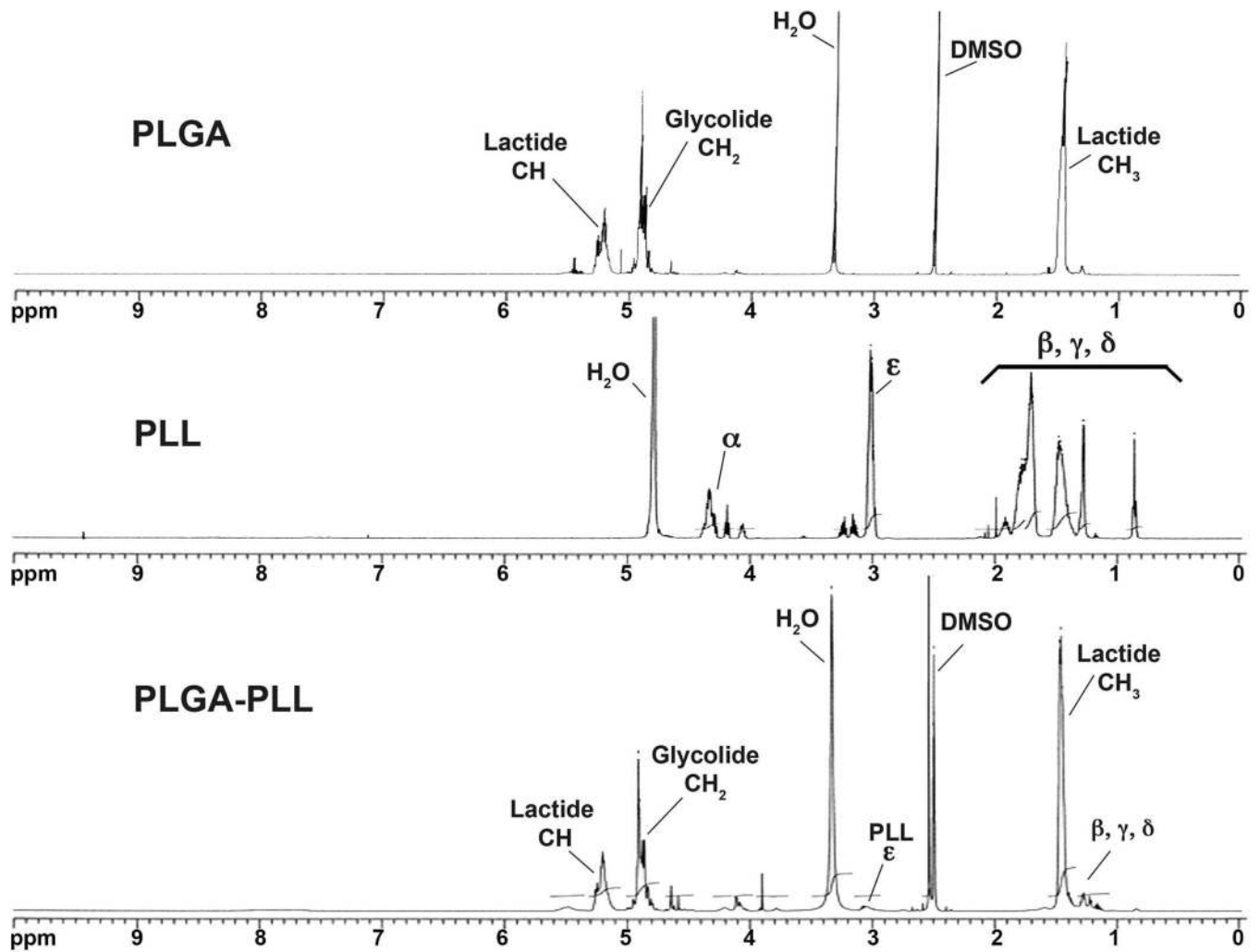
Figure 5. ^1\text{H-NMR} of PLGA, PLL and PLGA-PLL
