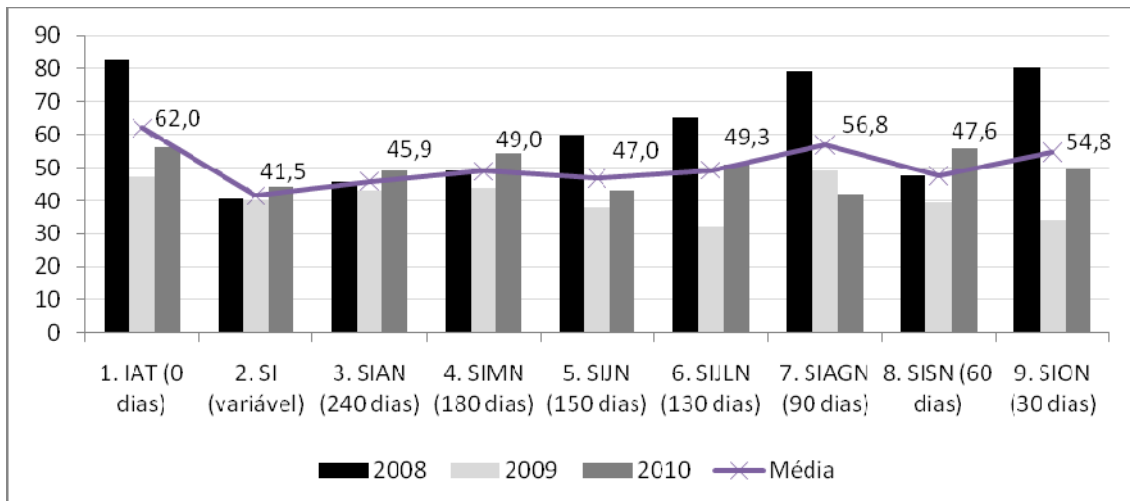
Figura 2: Produtividade média das safras de 2008 a 2010 dos diferentes tratamentos de irrigação, comparados com a testemunha não irrigada. Campo Experimental da Capal, Araxá, MG.
