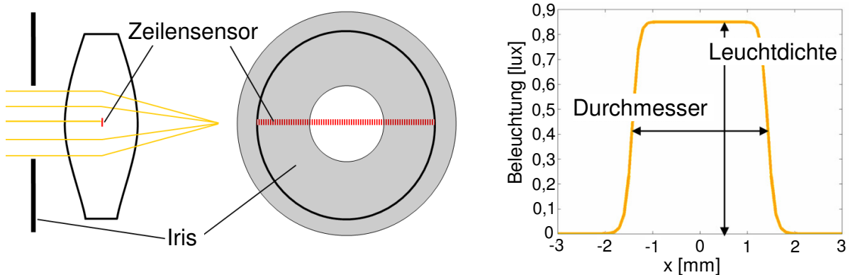
Abb. 2.9: Messung des Pupillendurchmessers und der Umfeldleuchtdichte zur Erfassung des Akkommodationsbedarfs (nach [Kli08]).
