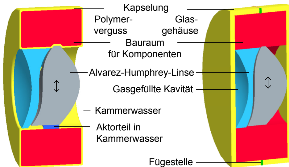
Abb. 3.23: Kapselungskonzepte für Alvarez-Humphrey-Linse: Polymerverguss mit Linse in Kammerwasser (links) und Glasgehäuse mit Linse in Gas (rechts) [RSGB09].
