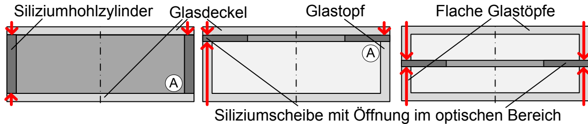
Abb. 3.17: Geometrievarianten für die Fertigung eines Gehäuses aus einem Siliziumbauteil (dunkelgrau) und zwei Glasbauteilen (hellgrau). Fügen durch Laserbonden ↓, Fügen durch anodisches Bonden (A). Schematische Schnittansichten.
