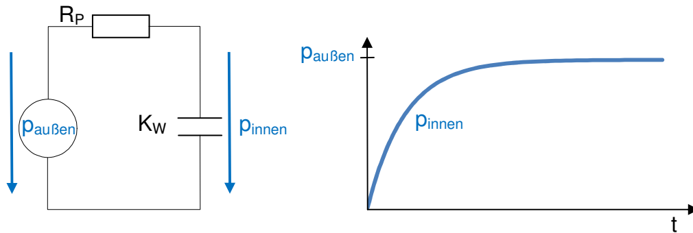
Abb. 4.3: Kondensatormodell für die Beschreibung des Anstiegs des Wasserdampfpartialdrucks p_{\text{innen}} in einem System in Abhängigkeit der Wasseraufnahmekapazität der internen Komponenten K_W , des Permeationswiderstands R_P des Gehäuses sowie des äußeren Wasserdampfpartialdrucks p_{\text{außen}}
