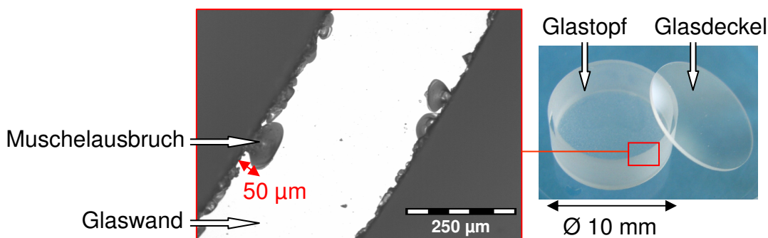
Abb. 5.7: Draufsicht auf eine mit Ultraschallbearbeitung gefertigte Borosilikatglaswand mit Muschelausbrüchen von maximal tolerierbarer Ausdehnung (links). Glasstumpf mit -deckel (rechts).
