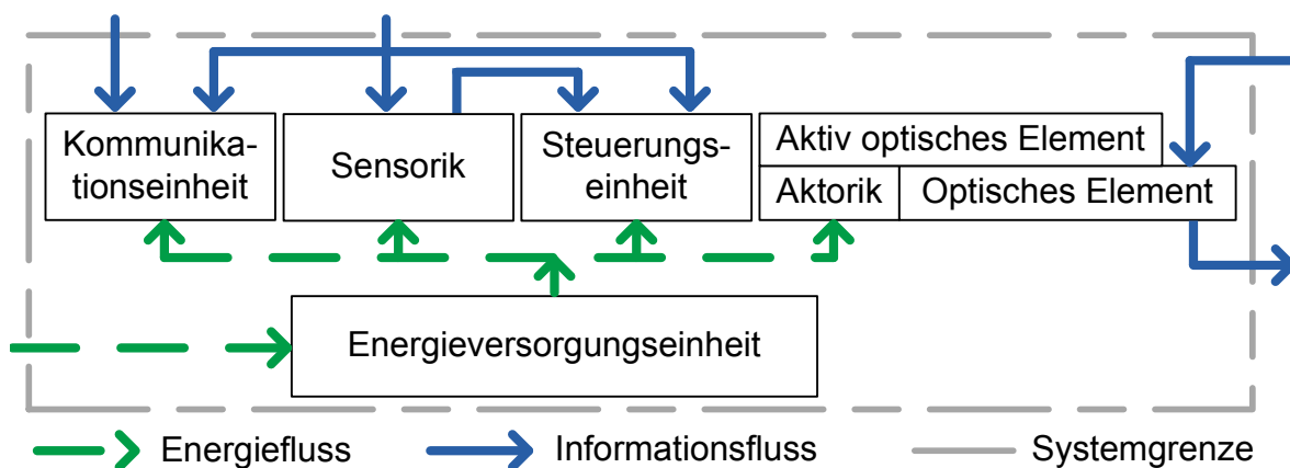
Abb. 2.5: Subsysteme und deren Energie- und Informationsflüsse im Künstlichen Akkommodationssystem (nach [Nag11]).
