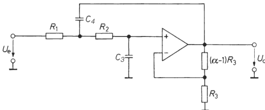
Abb. A.8: Aktives Tiefpassfilter zweiter Ordnung mit Einfachmitkopplung als Sallen-Key-Beschaltung [TS99].
