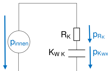
Abb. 4.4: Modell eines wasserabsorbierenden Körpers im Inneren eines Systems, in dem der Wasserdampfpartialdruck p_{\text{innen}} vorherrscht. Der Körper wird modelliert mit Hilfe des Vorwiderstands R_K und der Wasseraufnahmekapazität K_{WK} .
