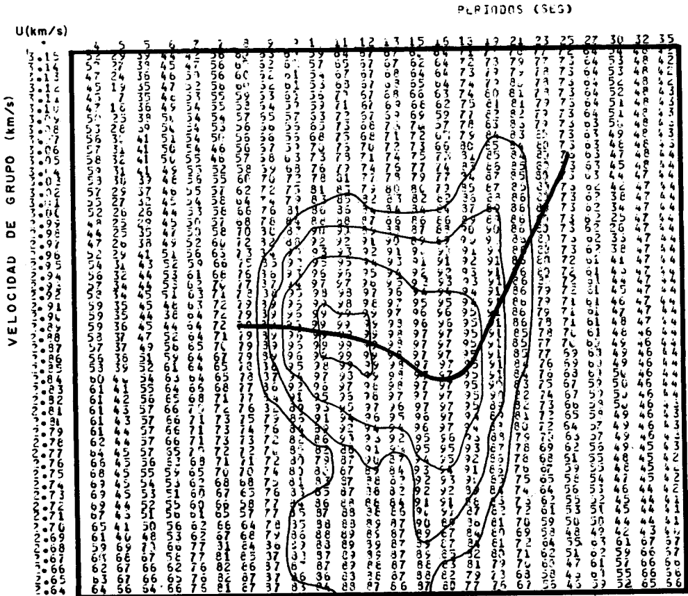
Fig. 4. Curva experimental de la dispersión de la velocidad de grupo para la explosión ZAZA (1967).
