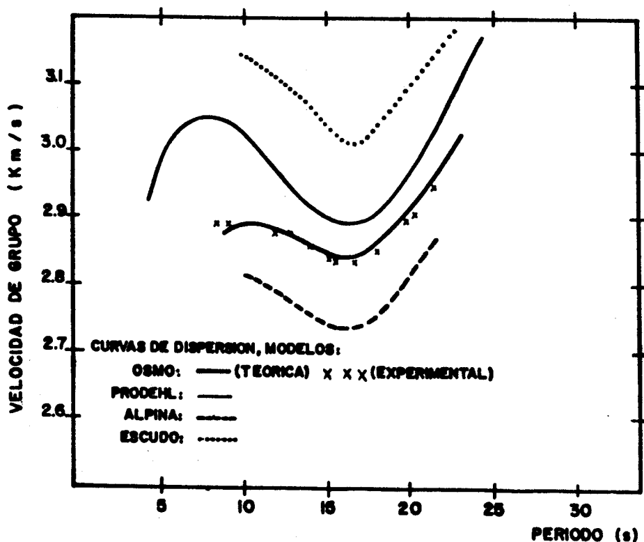
Fig. 10. Curvas de dispersión de la velocidad de grupo para el modo fundamental de las ondas superficiales de Rayleigh para los modelos OSMO, Nevada-Kingman, (Prodehl, 1979), y estructuras típicas Alpina y Escudo (Knopoff, 1966 y Brune, 1969) en comparación con los datos obtenidos para el perfil NTS-D.F.
