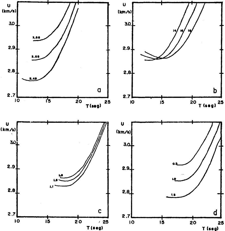
Fig. 3. Algunas curvas maestras usadas en este trabajo. Las gráficas a y b muestran los efectos sobre la curva de dispersión de la velocidad de grupo cuando se varía la velocidad de cizalle V_s y el espesor de la capa "3" del modelo de Fix, de 3.48 a 3.68 km/s y de 14 a 18 km, respectivamente. Las gráficas c y d muestran los efectos cuando se varían los valores de la velocidad V_s de 1.1 a 1.9 km/s y el espesor de 0.5 a 1.5 km en la capa "1" del mismo modelo (Tabla 2).
