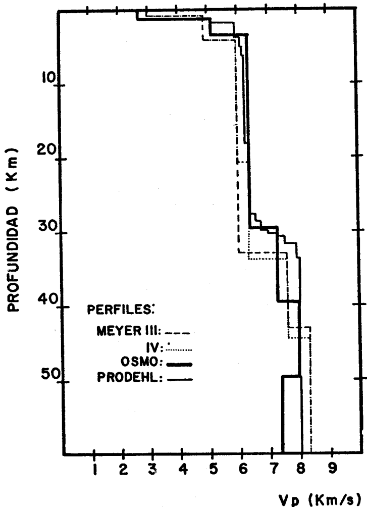
Fig. 9. Variación de la velocidad de las ondas longitudinales V_p con la profundidad, para los modelos OSMO, Nevada-Kingman (Prodehl, 1979), y núcleo de la Sierra Madre Occidental (Meyer y otros, 1961).
