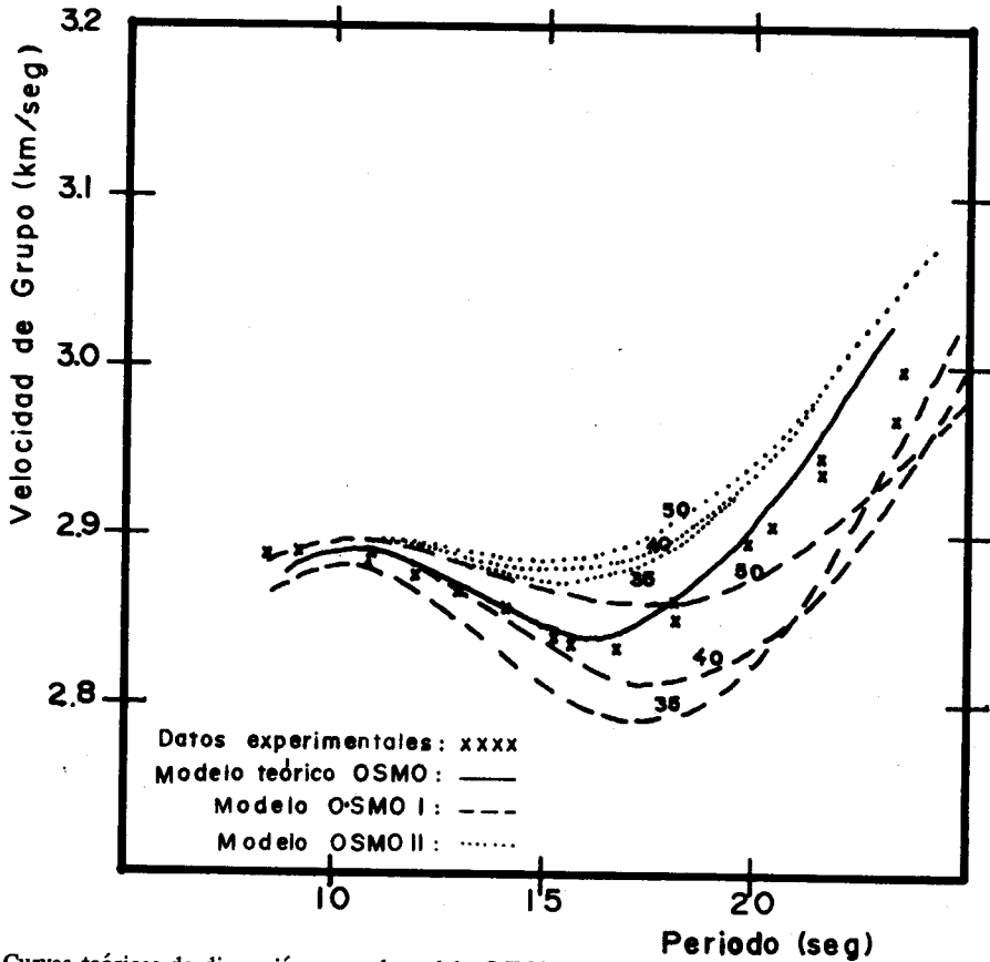
Fig. 7. Curvas teóricas de dispersión para el modelo OSMO y para los casos en que se elimine la región de baja velocidad del manto (OSMO I) o la región de alta velocidad de éste (OSMO II); los números asociados a cada curva teórica corresponden a los espesores totales de la corteza considerada, disminuyendo o incrementando el espesor de la capa basáltica. La curva que mejor ajusta los datos experimentales es la correspondiente al modelo OSMO (Tabla 3).
