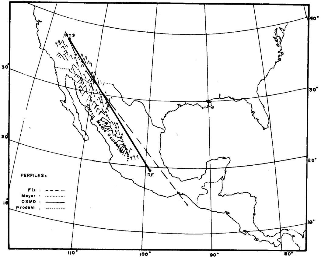
Fig. 1. Esquema de la localización del perfil estudiado (NTS-D.F.) que corre casi paralelo al oriente de la Sierra Madre Occidental. Se muestra la disposición geográfica de los perfiles estudiados por Meyer y otros (1958, 1961), Fix (1975) y Prodehl (1979). Perfiles cercanos a la región del presente estudio.
