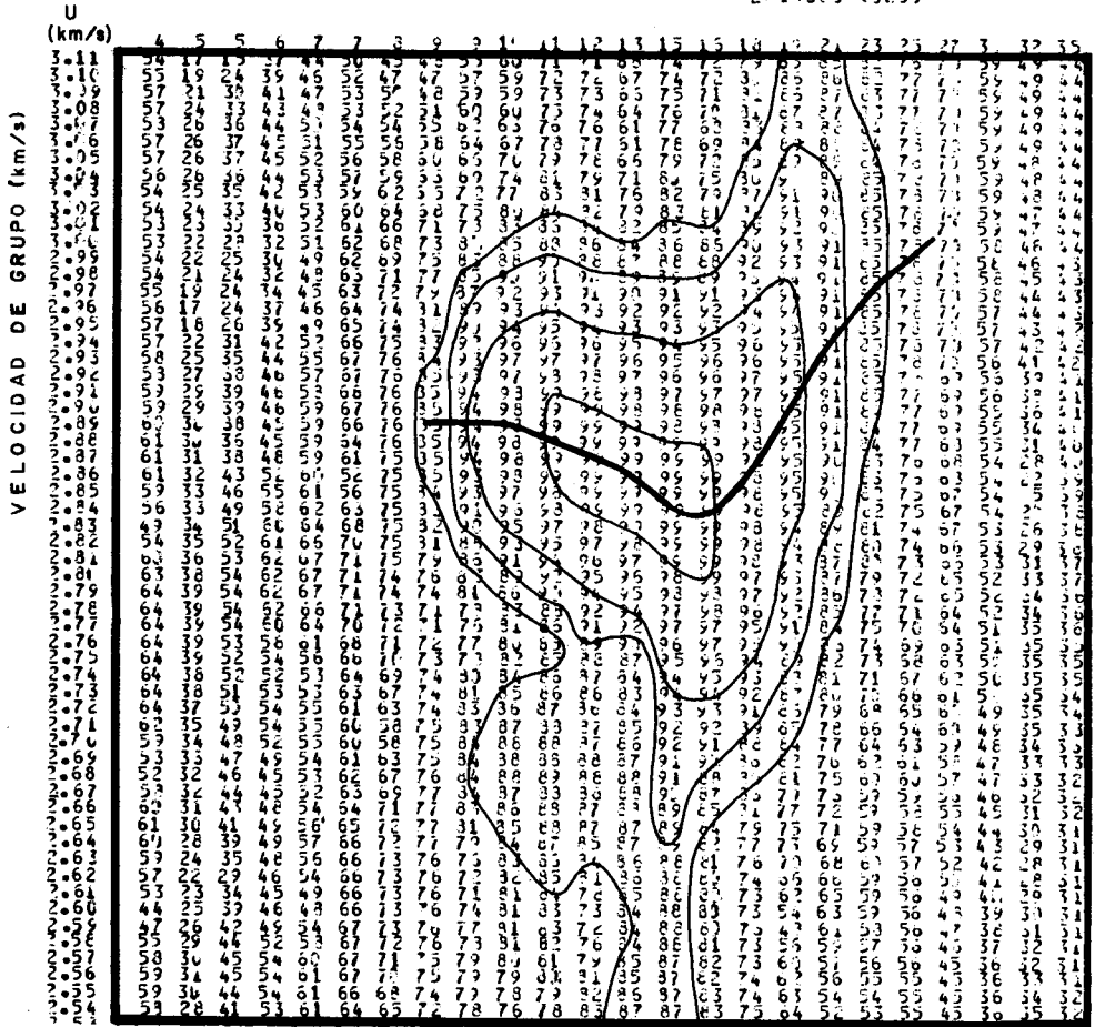
Fig. 5. Curva experimental de la dispersión de la velocidad de grupo para la explosión KNOX (1968).
