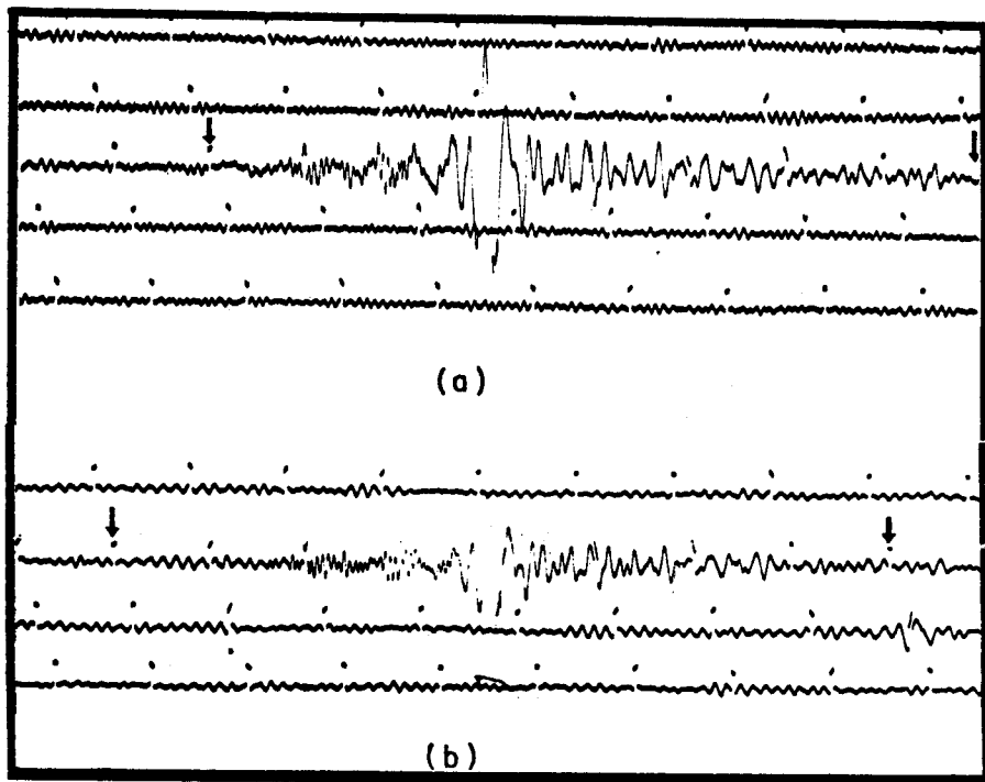
Fig. 2. Sismogramas correspondientes a las explosiones nucleares ZAZA (a) y KNOX (b), detonadas en el Sitio de Pruebas Nucleares en Nevada, USA en 1967 y 1968, respectivamente, y registradas en la estación UNM, México. Las flechas indican la porción del sismograma estudiado, que corresponde a una ventana de velocidades aparentes, comprendida entre 2.14 y 3.42 km/s.
