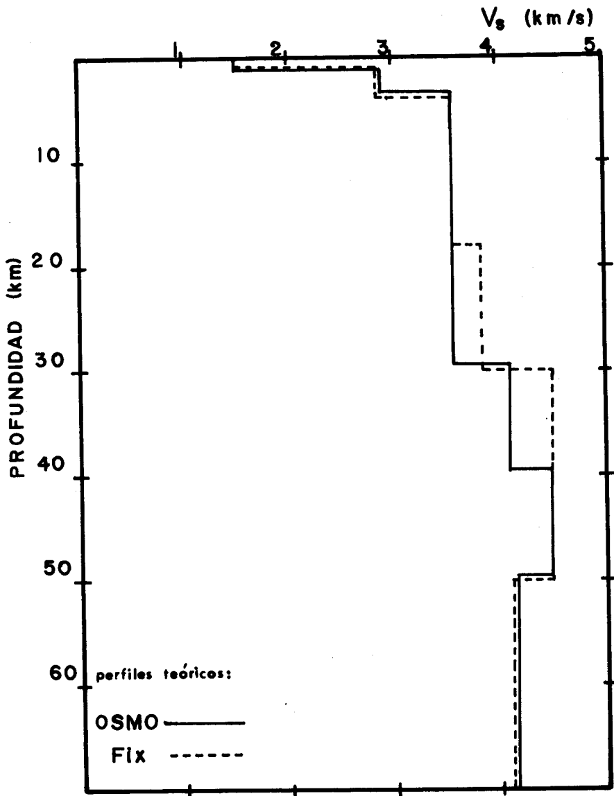
Fig. 8. Variación de la velocidad de las ondas de cizalle V_s con la profundidad, para los modelos: OSMO y Fix (1975).
