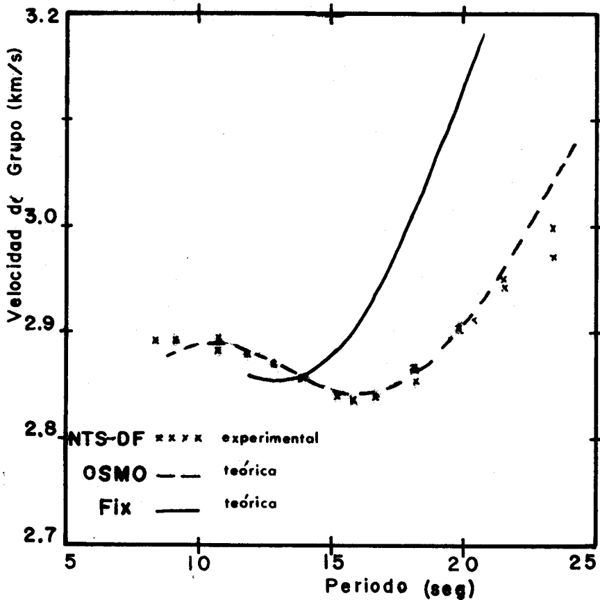
Fig. 6. Comparación entre las curvas experimentales de dispersión a lo largo del perfil NTS-D.F., la curva teórica correspondiente al modelo de capas para la corteza en la meseta central de México hallada por Fix (1975) y la curva teórica resultante del modelo OSMO obtenido en este trabajo (Tabla 3).
