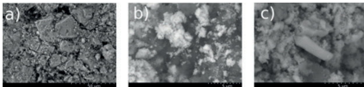
Figura 5. Imagen de electrones retrodispersados (BSE) de la capa de carbonato de plomo ( \text{PbCO}_3 ) en la munición Minié. El panel a) muestra una zona quebradiza correspondiente a los productos de Pb observados en la capa de la munición identificados como \text{PbCO}_3 con EDX a una resolución de 1000x. El panel b) y c) representan aumentos a 7000x y 9000x, respectivamente, de zonas de interés seleccionadas de a). El panel c) evidencia la aparición de una estructura periódica con forma y tamaño muy similar al cristal de cerusita \text{PbCO}_3 observada en investigaciones anteriores (elaboración propia).
