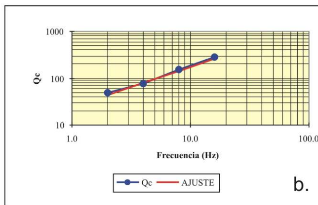
Figura 3. a) Valores de Qc obtenidos para todas las estaciones del campo geotérmico de Los Humeros como una función de la frecuencia. Los valores graficados son los valores promedio de Qc. b). Valores promedio de Qc para todo el campo geotérmico de Los Humeros y su respectivo ajuste (ver Tabla 2).
