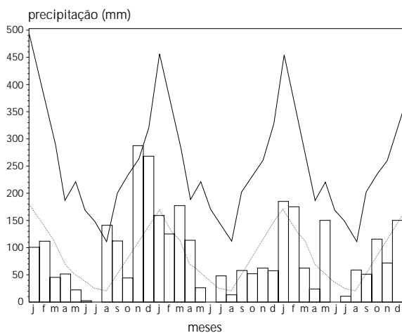
Figura 4 - Precipitação mensal em Corumbá, MS. Linha contínua: máxima do período 1925-1982; linha interrompida: média do período 1925-1982; retângulos: 1984-1986.
