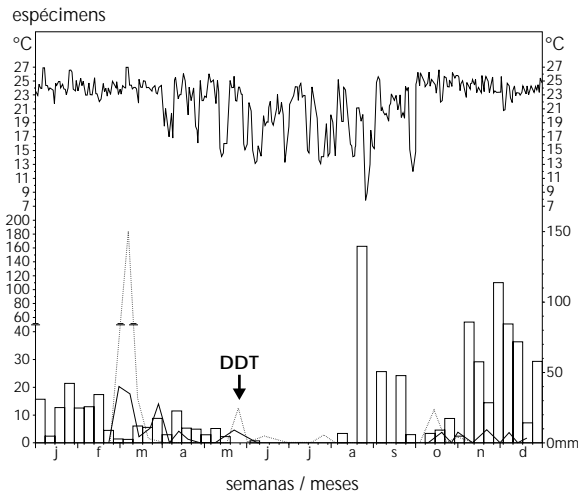
Figura 3 - Temperatura mínima diária e precipitação semanal no período de janeiro a dezembro de 1984. Número de flebotomíneos obtidos nas coletas semanais, nos peridomicílios dos bairros Centro (linha contínua) e Cristo Redentor (linha interrompida), no período de fevereiro a dezembro de 1984. A seta, indica a época de aplicação de inseticida. Município de Corumbá, MS.
