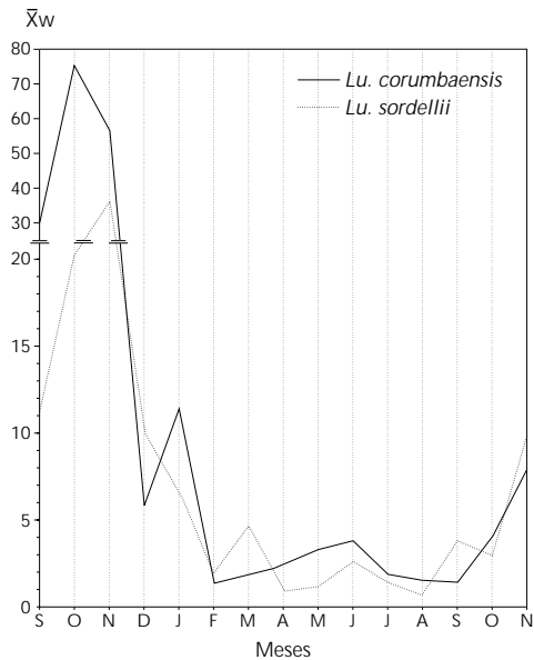
Figura 2 - Média de Williams ( \bar{X}_w ) mensal das espécies de flebotomíneos mais frequentes na gruta, para o período de maior regularidade das coletas, setembro/1984 a novembro/1985. Município de Corumbá, MS.
