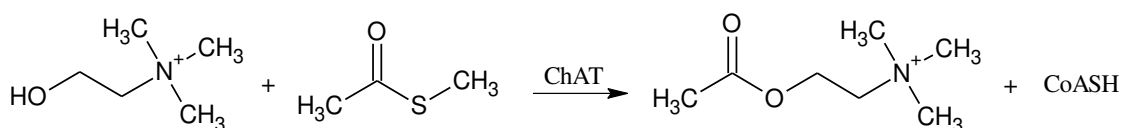
Figura 1.11 – Reação de biosíntese do neurotransmissor acetilcolina, adaptado de [52] .
