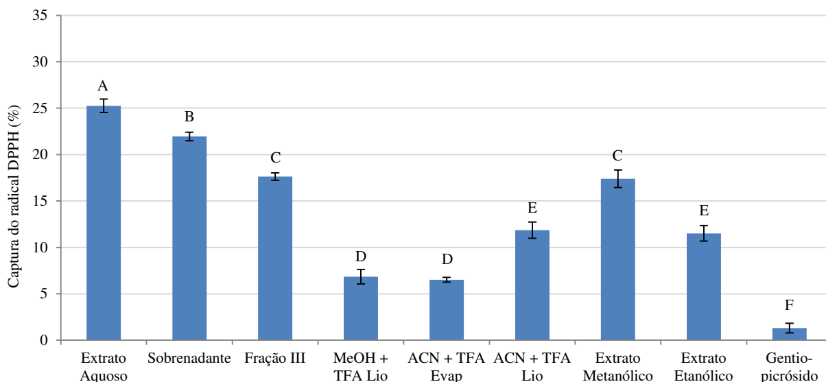
Figura 4.19 – Percentagem de atividade antioxidante, pela captura do radical DPPH, para as diferentes amostras, na concentração final de 50 \mu\text{g/mL} . Os padrões comerciais BHT, rutina e quercetina apresentam um \text{EC}_{50} ( \mu\text{g/mL} ) de 9,89 \pm 0,11 , 6,27 \pm 0,09 e 3,23 \pm 0,07 , respetivamente. Para um nível de confiança de 95 % A, B, C, D, E e F são estatisticamente diferentes.
