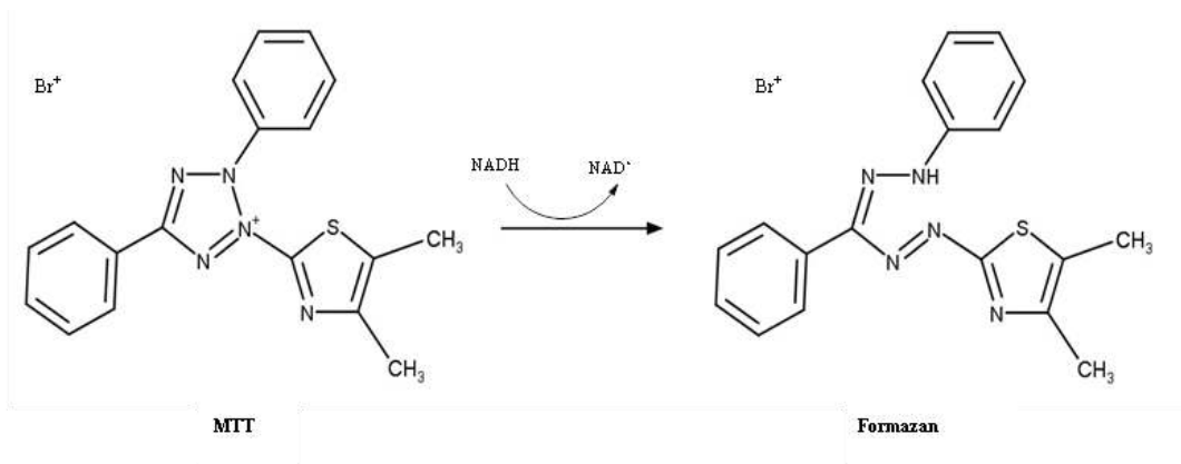
Figura 3.5 – Estruturas químicas do MTT e do seu produto reduzido formazan, adaptado de [84] .
