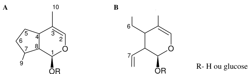
Figura 1.8 – Estrutura química do iridoíde (A), que sofre clivagem oxidativa e dá origem ao secoiridoíde (B), adaptado de [33] .
