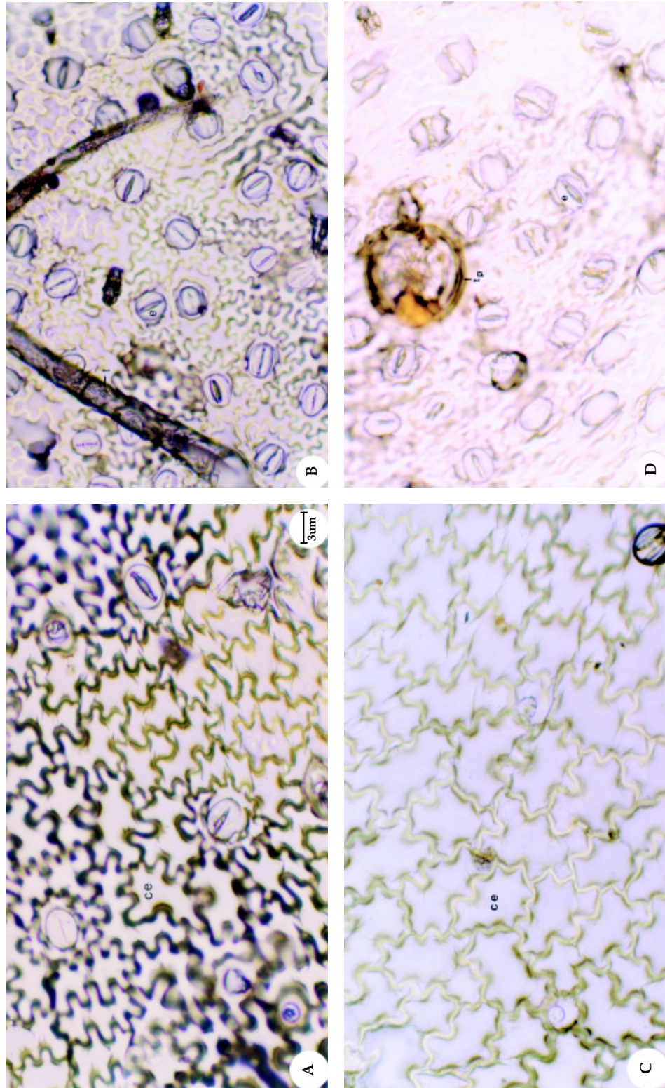
Figura 4. Seção paradérmica da lâmina foliar de Mentha spicata L. e de Mentha spicata X suaveolens . A: Epiderme adaxial de M. spicata (200x); B: Epiderme abaxial M. spicata (200x); C: Epiderme adaxial de M. spicata X suaveolens (200x); D: Epiderme abaxial M. spicata X suaveolens (200x). ce = célula epidérmica; e = estômato; tp = tricoma peltado.
