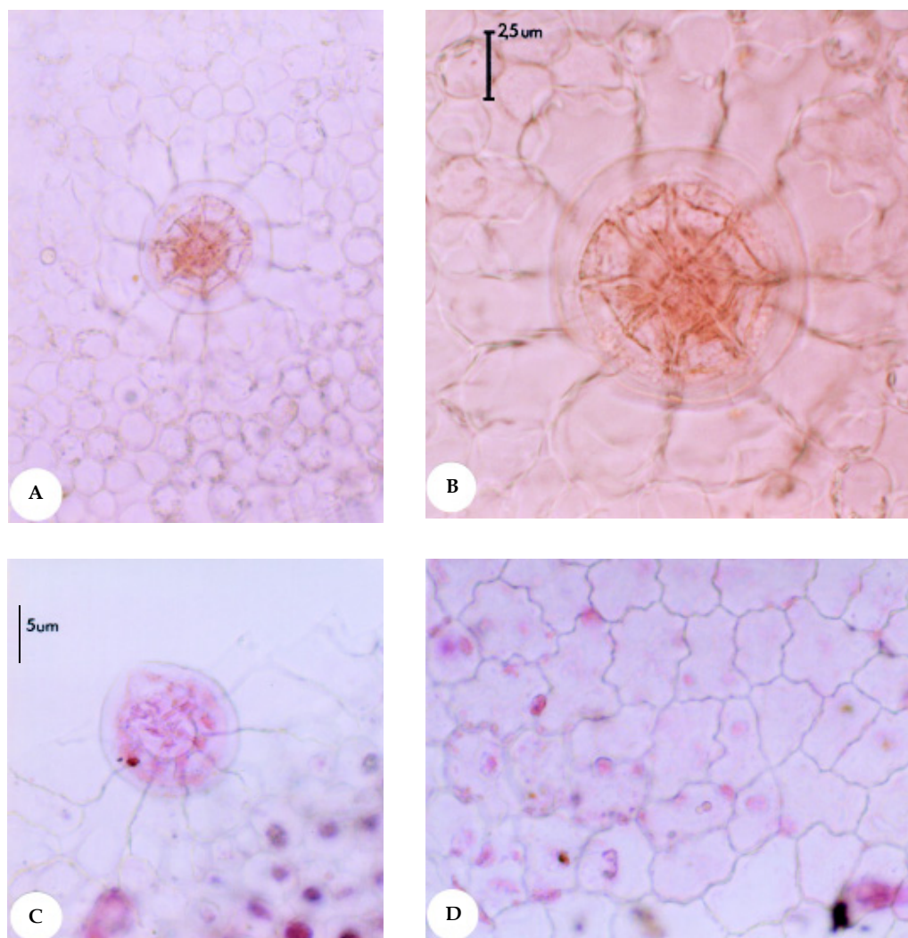
Figura 10. Secções paradérmicas da folha de Mentha spicata L. na face adaxial da epiderme. A: Tricoma peltado formado por 12 células secretoras, dispostas em dois círculos concêntricos. Detalhe do tricoma tector inserido na nervura principal da folha na face abaxial e (C) face abaxial da folha. B: Idem em detalhe (400x); C e D: Secções paradérmicas da folha de Mentha spicata X suaveolens na face adaxial de epiderme (200x). Tricoma peltado formado por 12 células secretoras, dispostas em dois círculos concêntricos, quatro células constituindo a coroa central e oito células circundando a coroa.
