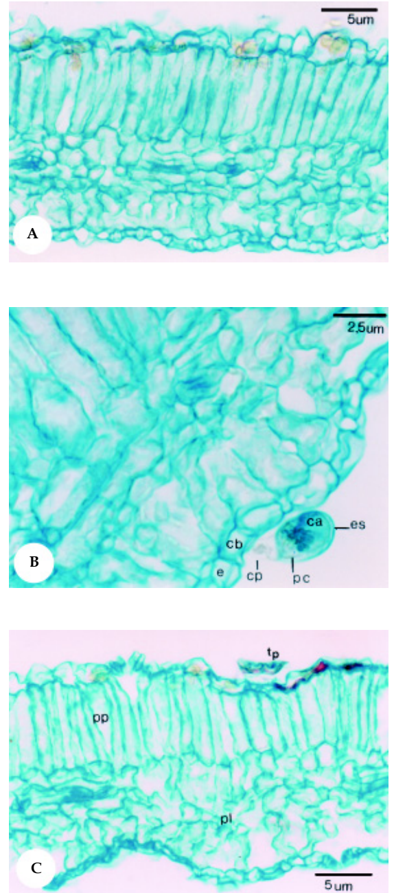
Figura 2. Secção transversal da lâmina foliar de Mentha spicata L. A: Corte transversal da lâmina foliar (200x); B: Detalhe de tricoma capitado do Tipo I (400x); C: Detalhe de tricoma peltado (200x). e = epiderme; pp = parênquima paliçádico; pl = parênquima lacunoso; cb = célula basal; cp = célula peduncular; ca = célula apical; es = espaço subcuticular; tp = tricoma peltado; pc = parede celular.
