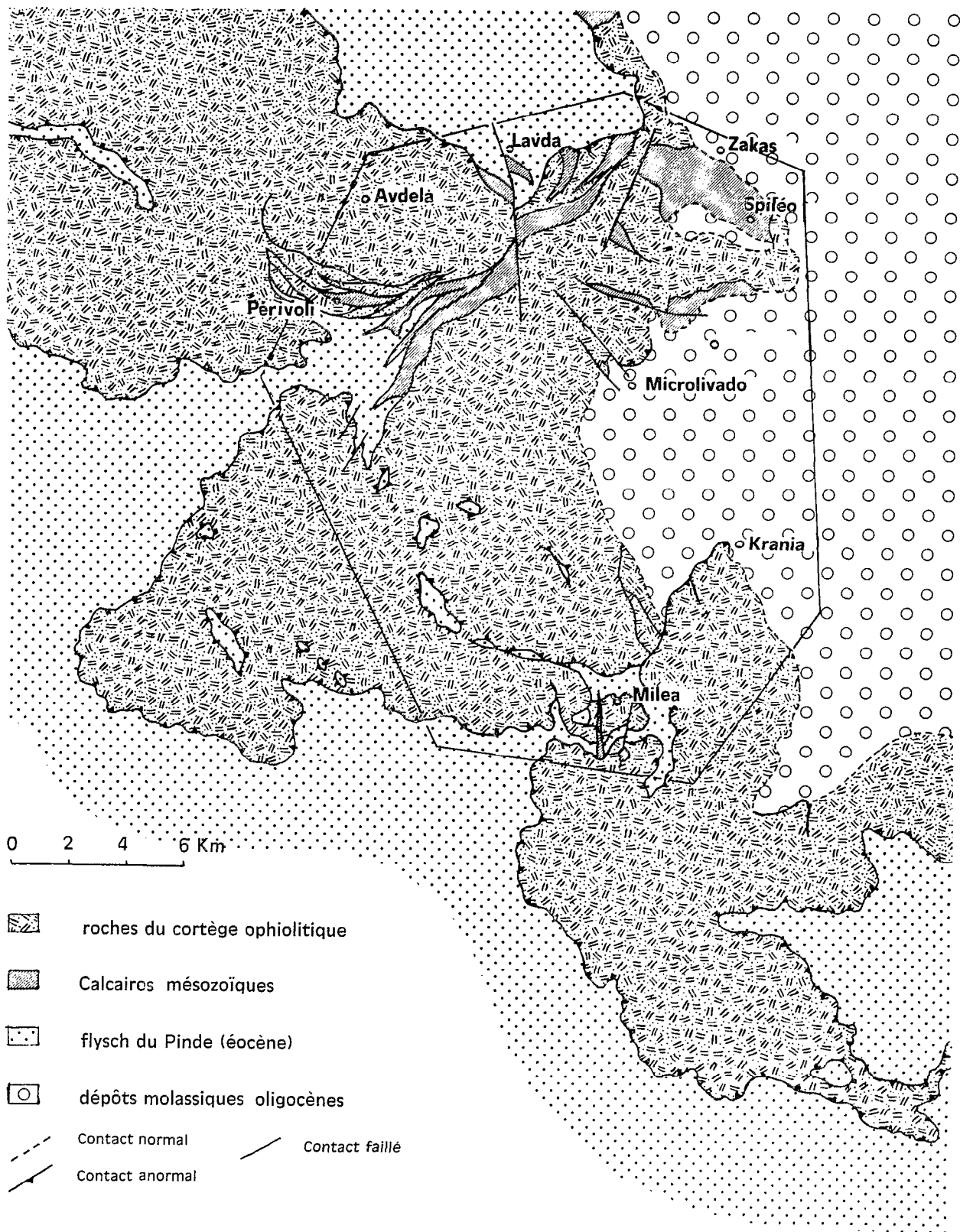
FIG. 2. — Le Massif ophiolitique du Pinde septentrional et le secteur étudié (cf. carte H.T.).
