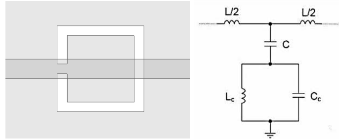
Fig. II. 14. La ligne de transmission chargée du RAFC et son modèle de circuit équivalent.
