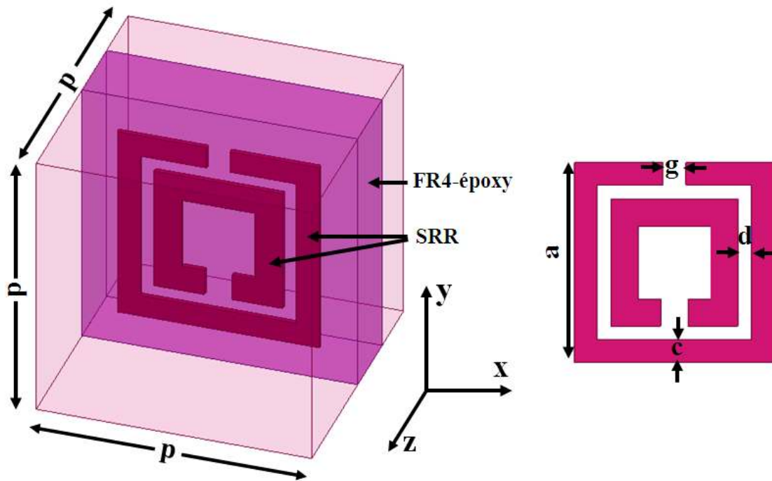
Fig. II. 7. Représentation et paramètres d'une unité de cellule du RAF carré.
