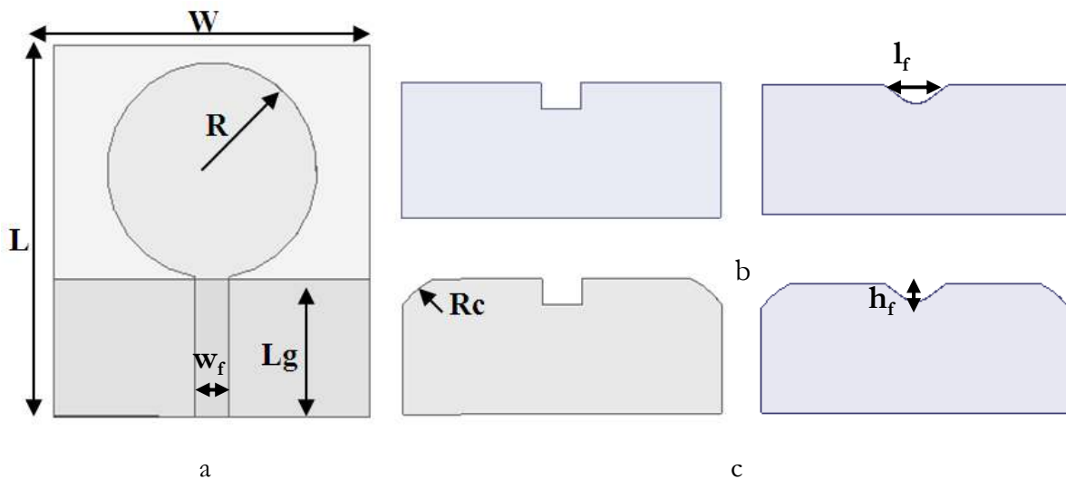
Fig. III. 1. Etapes de conception de l'antenne : (a) étape_1. (b) étape_2. (c) étape_3.
