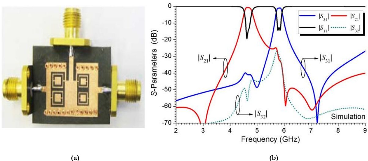
Fig. I. 27. (a) Duplexeur SIW- RAFC. (b) le coefficient de transmission et d'isolation [56].
