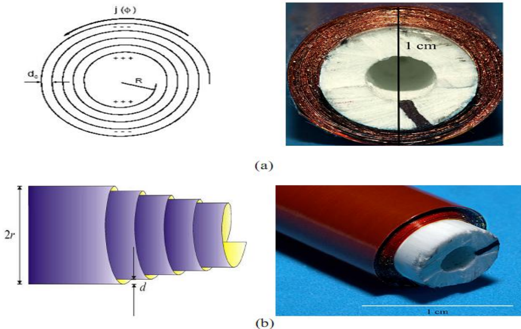
Fig. I. 2. Structure de rouleau suisse introduite par Pendry :
