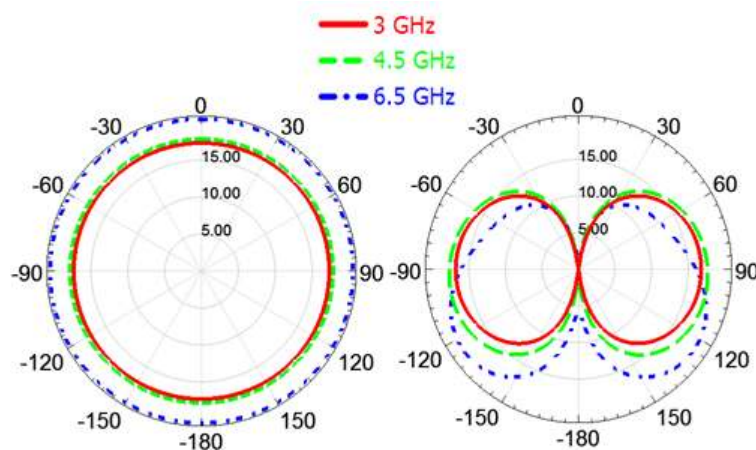
Fig. A. 6. Diagramme de rayonnement pour le Plan H (à droite) et le plan E (à gauche).
