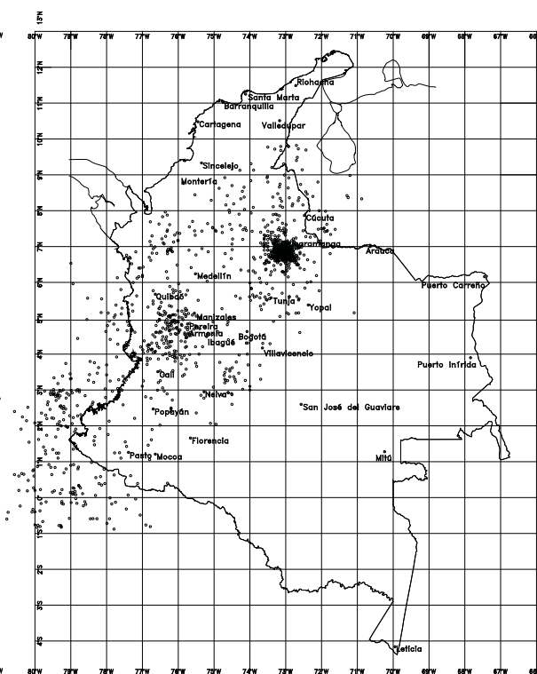
Figura 4. Eventos asignados a fuentes profundas
