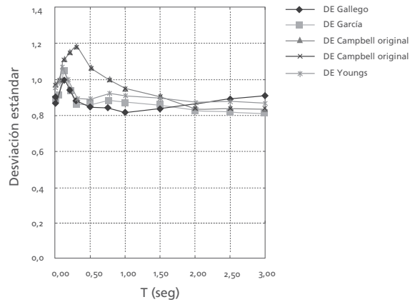
Figura 10. Comparación desviaciones estándar zona de Benioff
