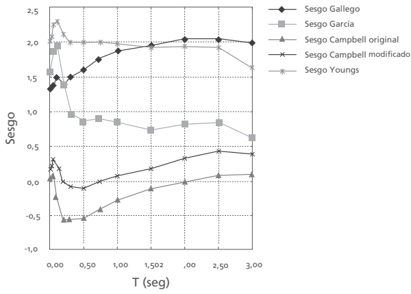
Figura 7. Comparación sesgos zona subducción
