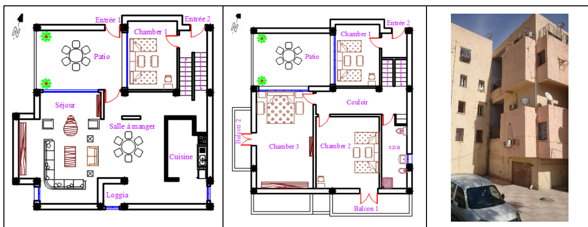
Fig.7. Plans et façade du logement
