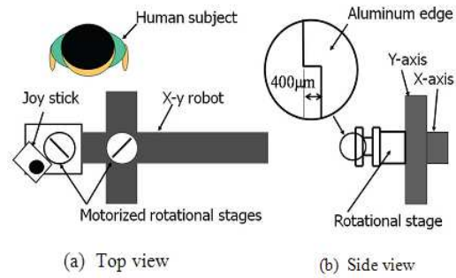
Fig. 1: Real edge presentation apparatus
