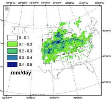
Low ET Years: 1990, 2002, 2006
