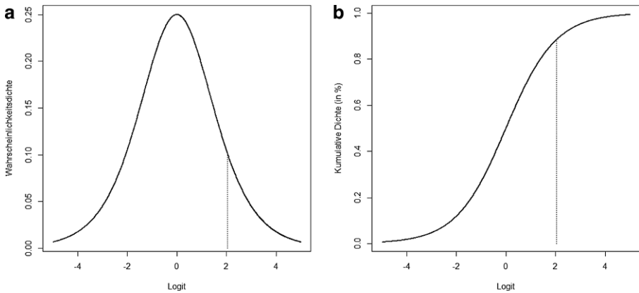
Abb. 6 Darstellung der Dichte der standard-logistischen Verteilung (a) auf welcher die Kategoriengrenzen der ordinalen Regression aufgetragen werden sowie der resultierenden kumulativen Dichte (b). In gestrichelter Linie ist exemplarisch eine Kategoriengrenze mit einem Logit von 2.04 aufgetragen
