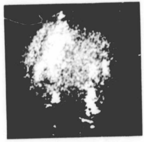
Ca II 3933
