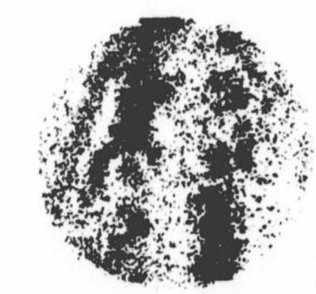
Mg x 625
