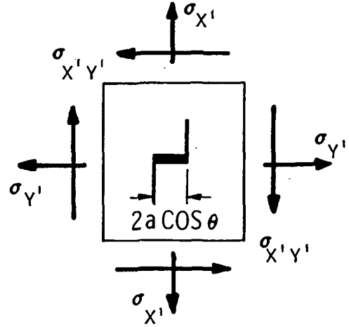
(d) EQUIVALENT AXIAL NOTCH
