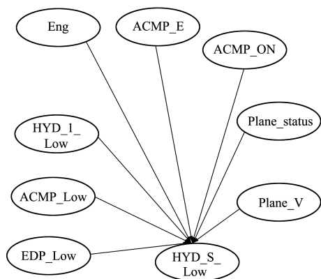
图 2 1号液压系统低压故障贝叶斯网络
