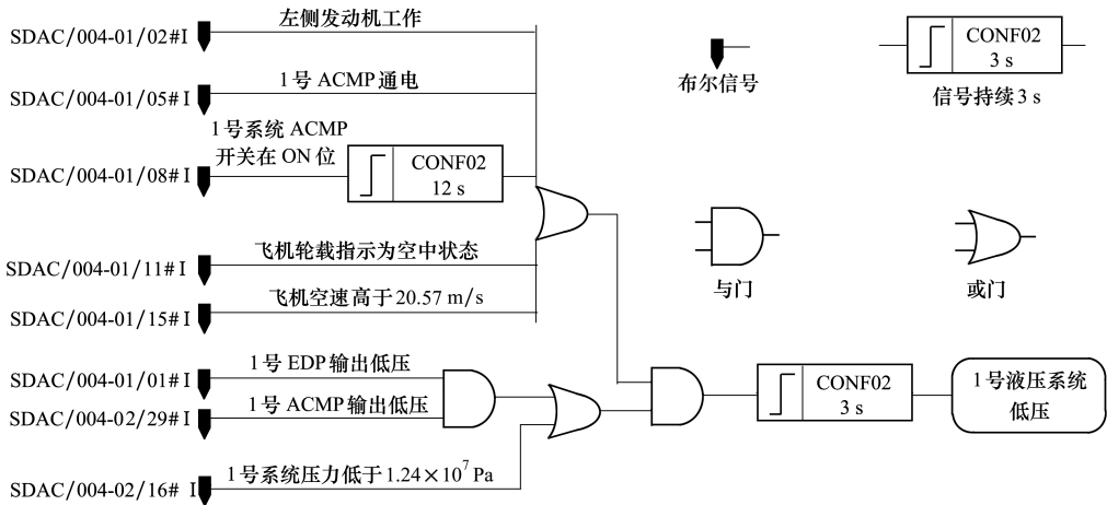
图 1 1号液压系统低压故障逻辑图
