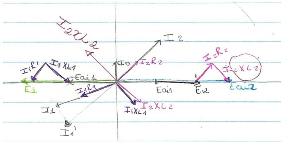
Figura 1 – Diagrama vetorial do transformador real com carga.
