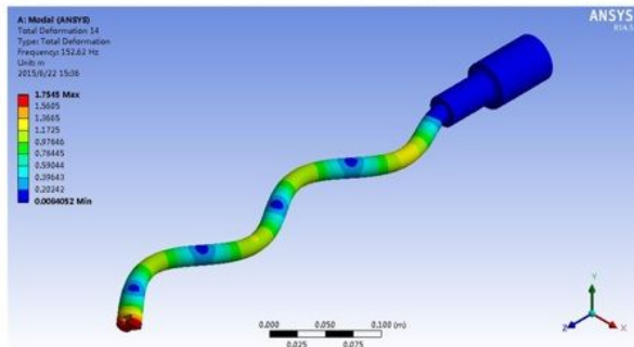
(d) Vibration mode at the frequency of 152.62Hz
