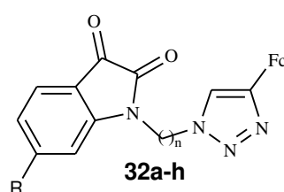
32a: R= H; 32b: R= F; 32c: R= CH 3 ; 32d: R= Cl n = 2 32e: R= H; 32f: R= F; 32g: R= CH 3 ; 32h: R= Cl n = 3
