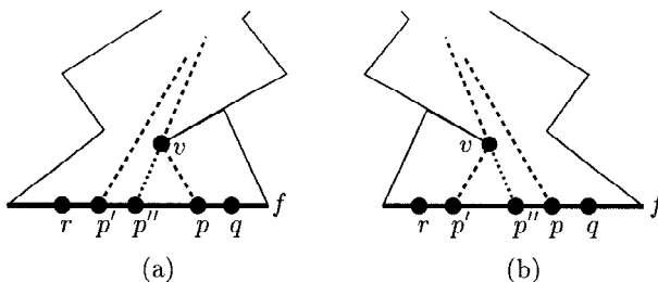
Fig. 8. Illustrating Lemma 4.4.
