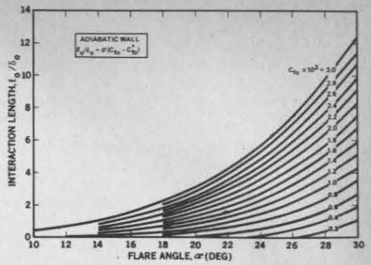
Fig. 9 Upstream influence due to a flare.
