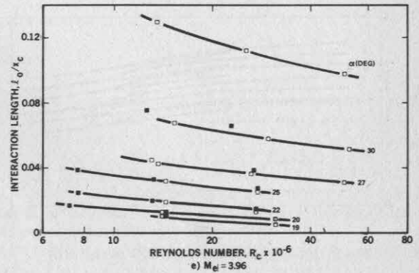
e) M_e = 3.96
