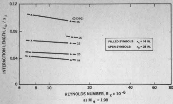
a) M_e = 1.98
