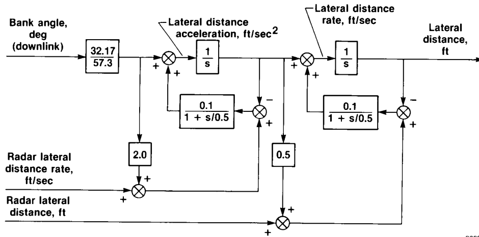
(d) Lateral distance calculation.
