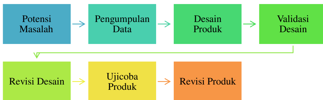
Gambar 1. Desain Penelitian
