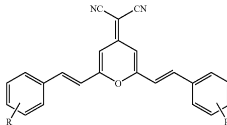
Pyran
