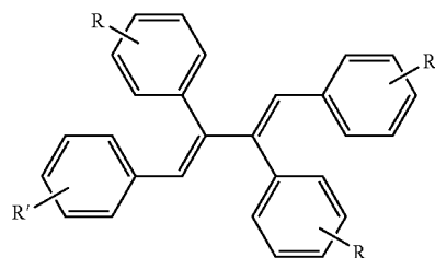
Butadiene
