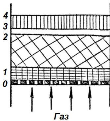
Рис. 3 – Зони газорідного шару на решітці. 0 - 1 зона пінно-струменевої; 1 - 2 зона пінного шару; 2 - 3 зона піни підвищеної щільності; 3 - 4 зона бризок
