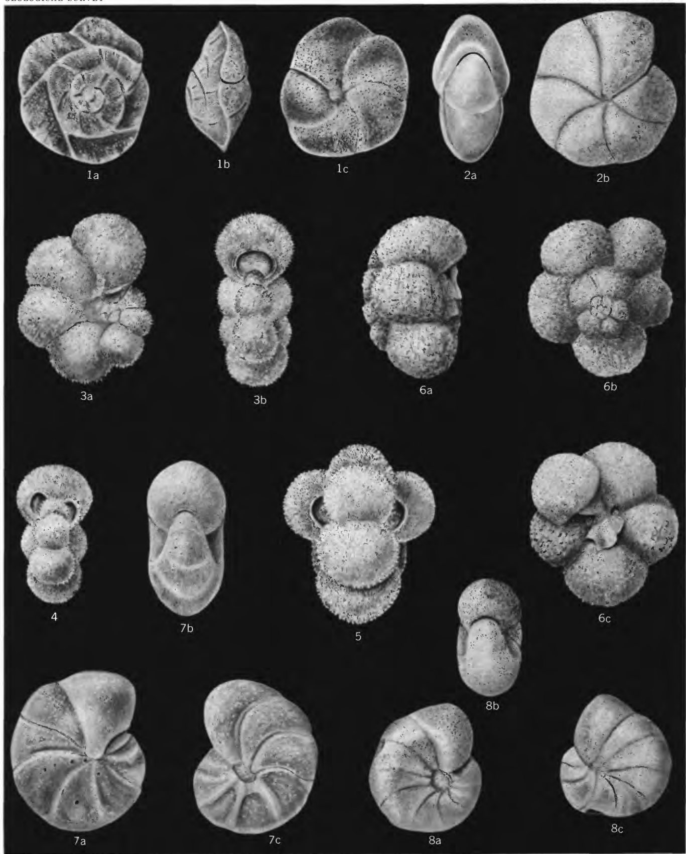
NUTTALLINELLA? , PULLENIA , BIGLOBIGERINELLA , RUGOGLOBIGERINA , AND ANOMALINOIDES
