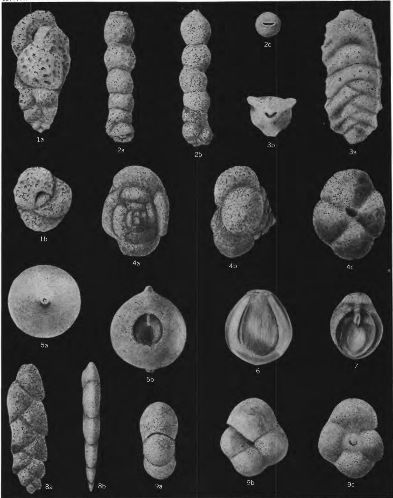
VERNEULINOIDES, PSEUDOCLAVULINA?, CLAVULINOIDES, TROCHAMMINA OOLINA, FISSURINA, ?LOXOSTOMA, AND "DISCORBIS"
