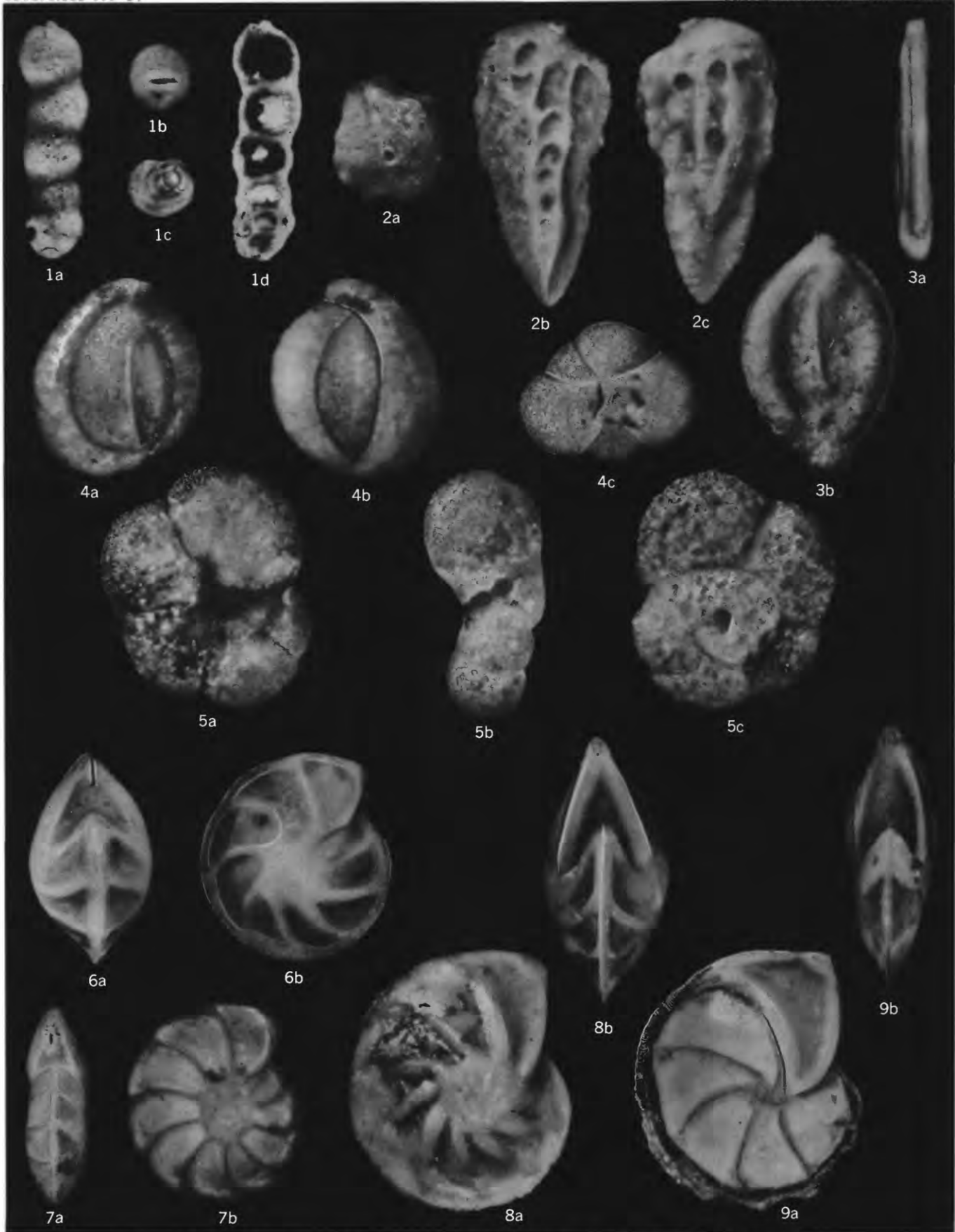
PSEUDOCLAVULINA? , HETEROSTOMELLA , SILICOSIGMOILINA , QUINQUELOCULINA , TROCHAMMINA , AND ROBULUS
