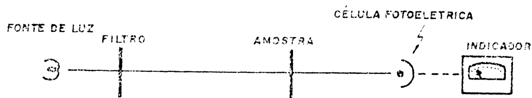
Figura 1 — Esquema de um densitômetro de transmissão.
