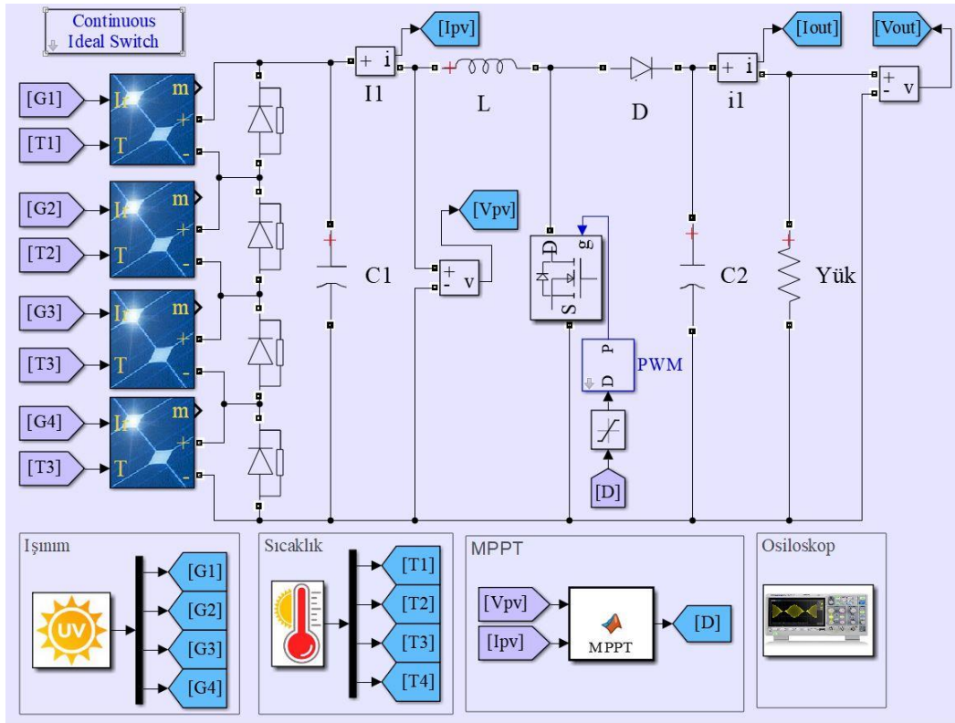
Şekil 9. Sistemin MATLAB/SIMULINK modeli (MATLAB / SIMULINK model of the system)
