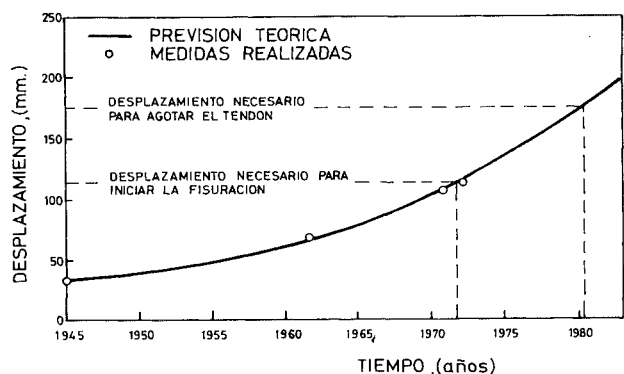
Fig. 21.—Evolución del desplazamiento máximo de la coronación.
