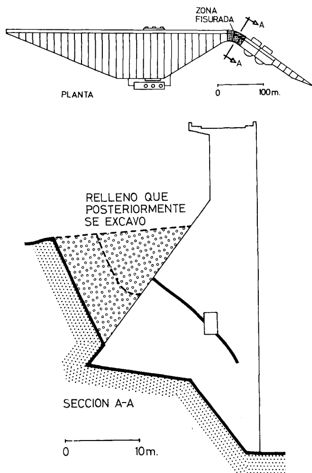
Fig. 13.—Planta y sección, por el codo, de la presa de Fontana.
