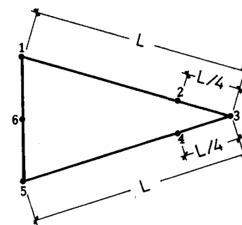
Fig. 3.—Triángulos isoparamétricos de seis nudos.
