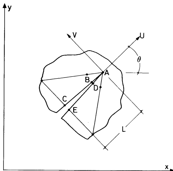
Fig. 4.—Elementos singulares que rodean el fondo de una fisura.
