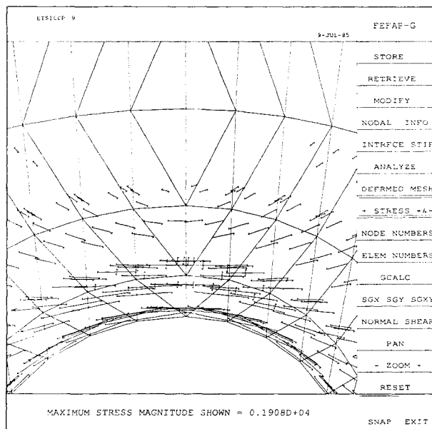
Fig. 10.—Dirección y magnitud de las tensiones máximas.
