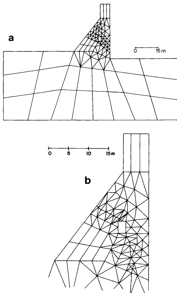
Fig. 17.—Malla de elementos finitos utilizada para estudiar la propagación de la fisura: a) Malla inicial, b) Malla final.
