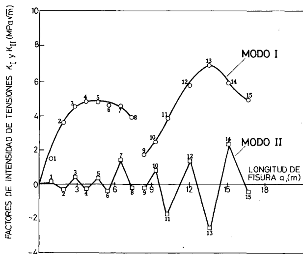
Fig. 19.—Valores de los factores de intensidad de tensiones, después de cada incremento de la fisura.
