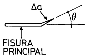
Fig. 5.—Fisura desviada. Notación.
