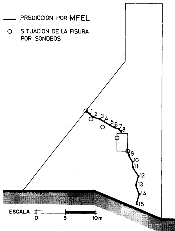
Fig. 20.—Propagación de la fisura, comparación entre las predicciones teóricas y los sondeos.
