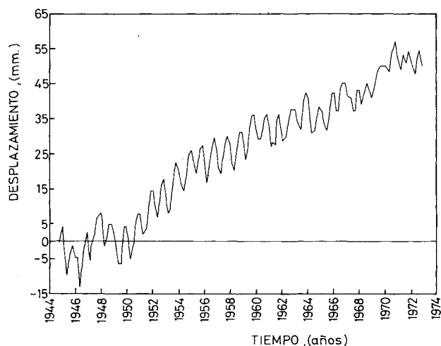
Fig. 16.—Registros de los desplazamientos de la coronación.
