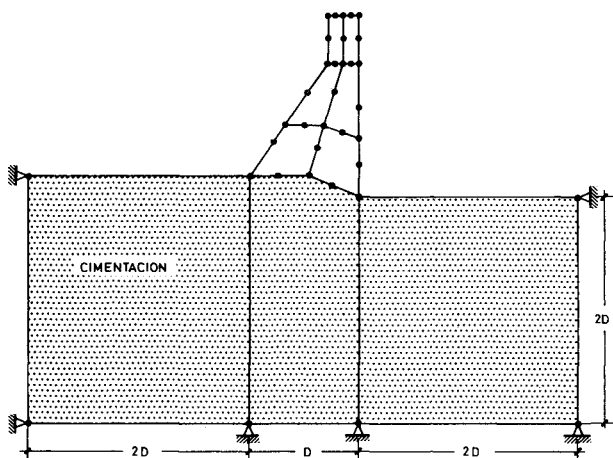
Fig. 14.—Sección de la malla de elementos finitos tridimensionales en la región del codo.
