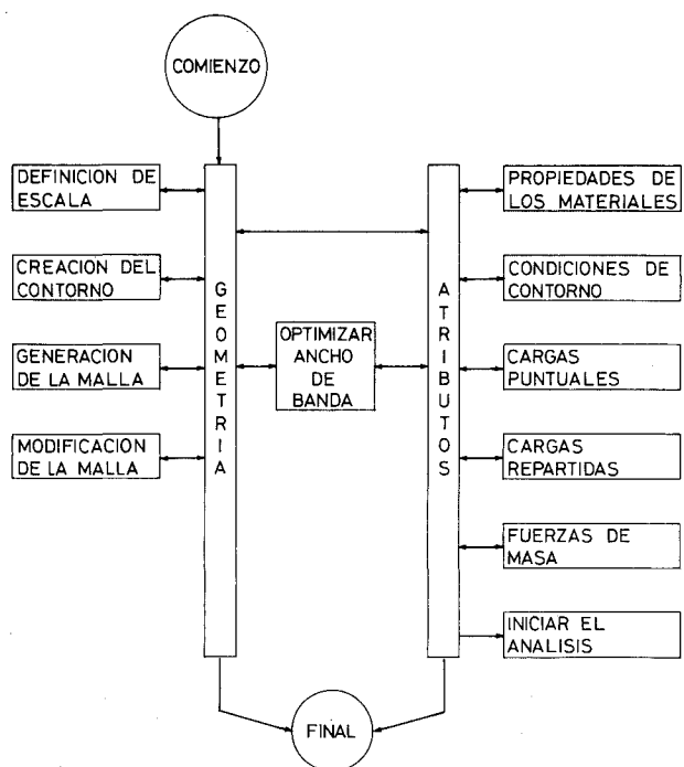
Fig. 7.—Diagrama de flujo del preproceso.
