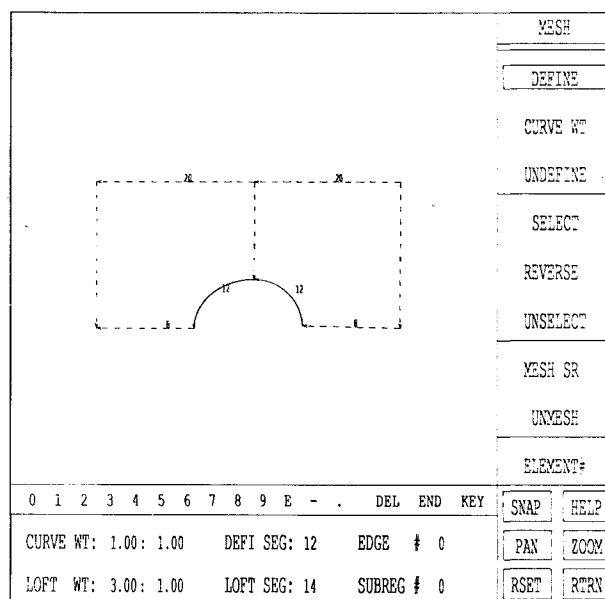
Fig. 8.—Generación de mallas. Selección de nudos en el contorno.
