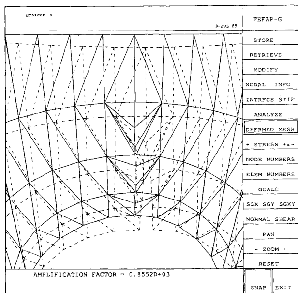
Fig. 12.—Malla fisurada y deformada de la estructura.
