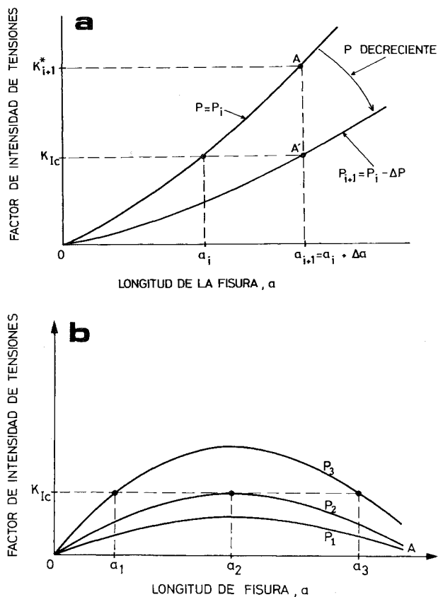
Fig. 6.—Variación del factor de intensidad de tensiones para el caso 1 (a) y para el caso 2 (b).
