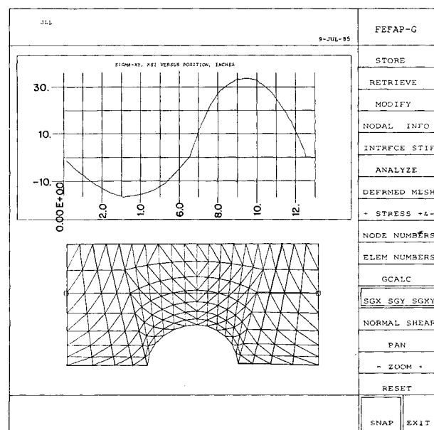
Fig. 11.—Variación del estuerzo cortante a lo largo de la estructura.
