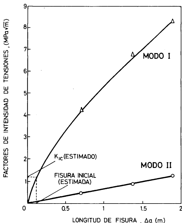
Fig. 18.—Estimación de la tenacidad de fractura del hormigón a partir de los factores de intensidad de tensiones y del tamaño estimado de la fisura inicial.
