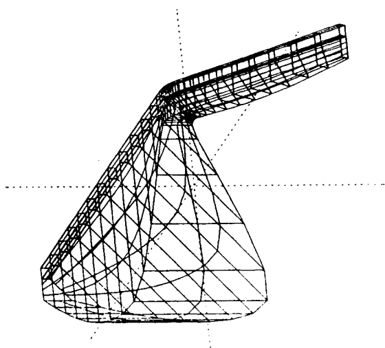
Fig. 1.—Presa de Fontana. Malla de elementos finitos tridimensionales.
