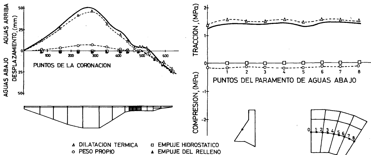
Fig. 15.—Resultados del cálculo tridimensional. Desplazamientos de la coronación y tensiones en el centro del paramento de aguas abajo.
