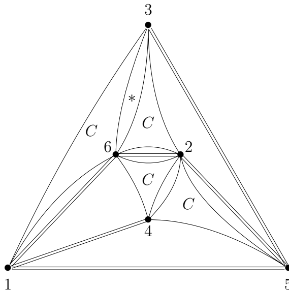
Fig. 1: \mathcal{H}'_{2,4}
