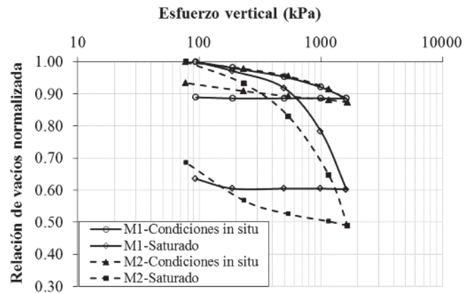
Figura 11. Curvas de compresibilidad normalizadas con respecto a la relación de vacíos. Ensayo doble-edómetro Fuente: el autor
