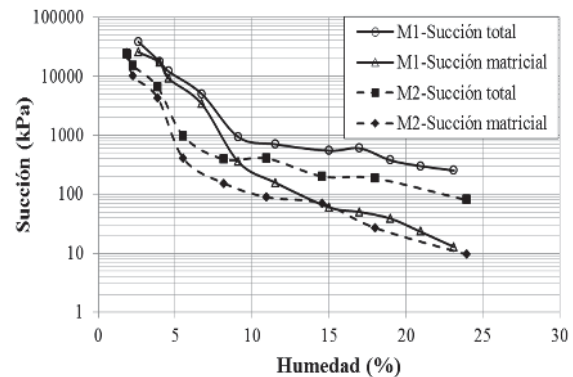
Figura 14. Curva característica del suelo. Succion total y matricial Fuente: el autor.
