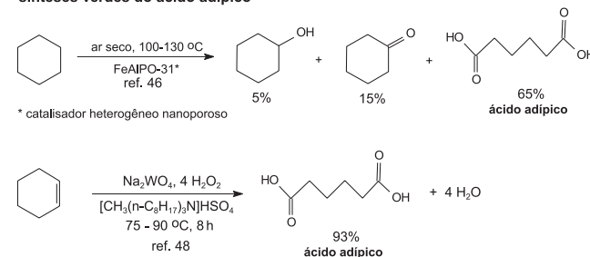
Figura 3. Métodos de obtenção do ácido adípico: processo industrial clássico e duas alternativas de síntese verde
