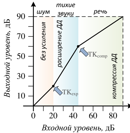
Рис. 9. Характеристика входа-выхода КДД
