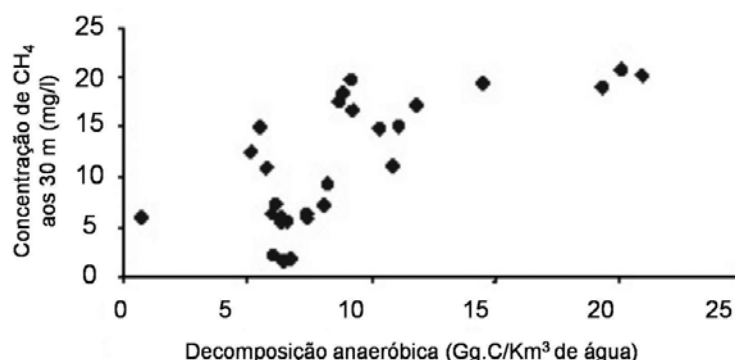
Figura 1. Concentração de metano ( \text{CH}_4 ) a 30m de profundidade contra carbono decomposto anaerobicamente. Dados de concentração a 30m são de Petit Saut (Galy-Lacaux et al. 1999), que é de Tucuruí (J.G. Tundisi, em Rosa et al. 1997).
