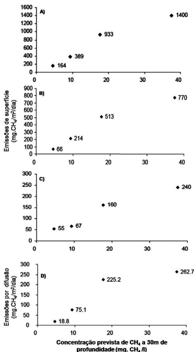
Figura 2. Borbulhamento e emissões de difusão contra concentração de metano prevista a 30m de profundidade. Dados de emissões são de Petit Saut (Galy-Lacaux et al. 1999). A.) Borbulhamento para locais 0-3m de profundidade; B.) Emissões de borbulhamento para 4-6m de profundidade; C.) Emissões de borbulhamento para 7-8m de profundidade; D.) Emissões de difusão para todas as profundidades.
