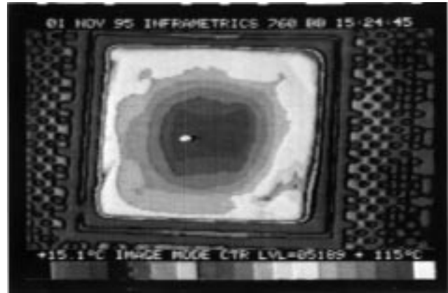
Fig. 18. 21164 thermal image.
