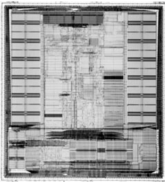
Fig. 3. 21164 die photo.
