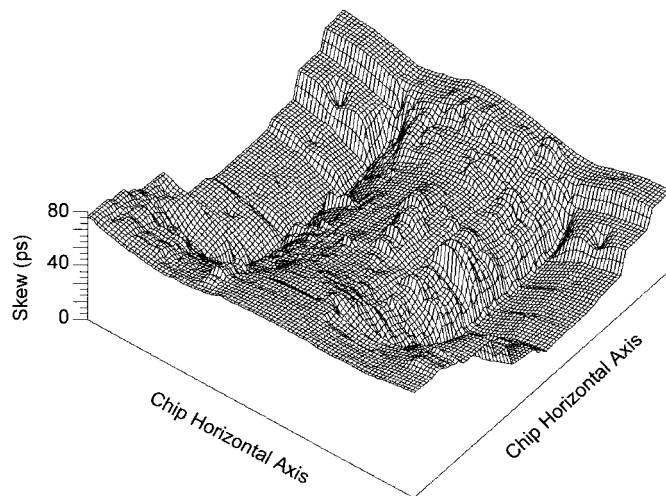
Fig. 17. 21164 clock skew.
