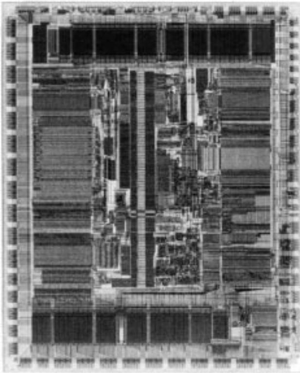
Fig. 2. 21064 die photo.
