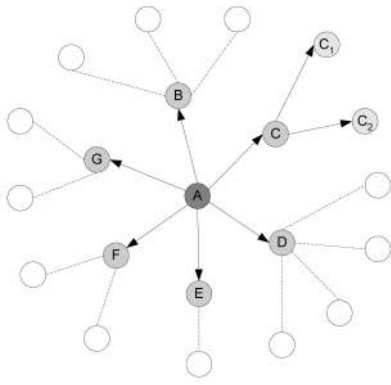
Fig. 2. Histogram update.
