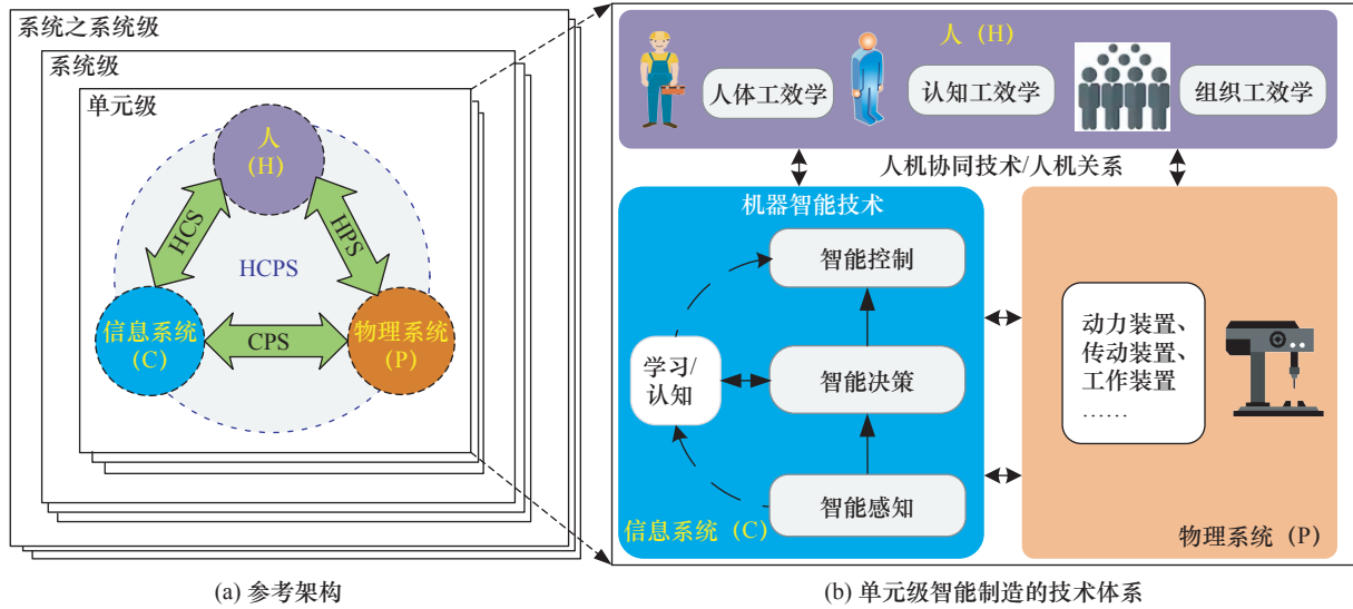
图 2 人本智造的技术体系示意图 [2, 3, 5] 注：HPS 表示人-物理系统；HCS 表示人-信息系统。
